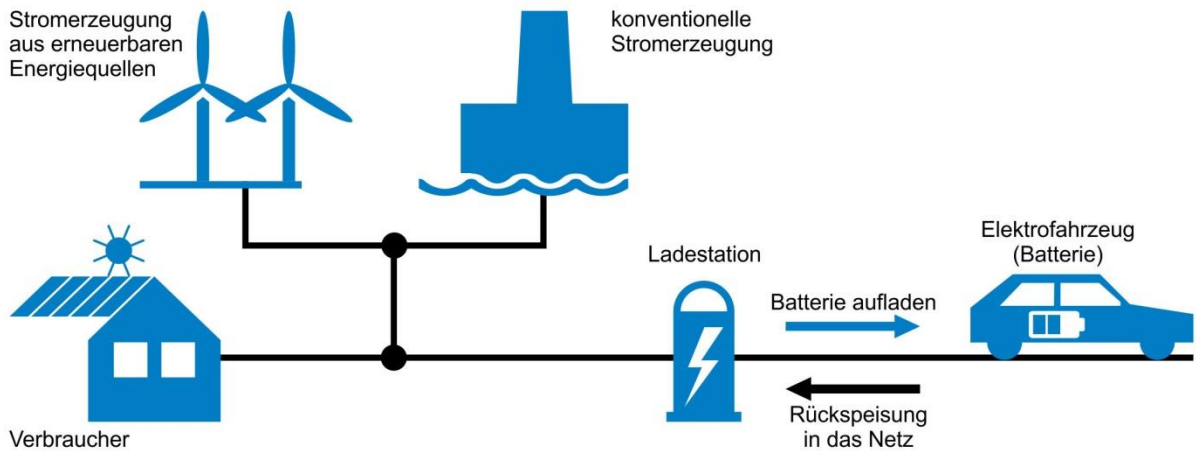
Abbildung 2 Schematische Darstellung einer bidirektionalen Ladung (Quelle: Wiener Netze)
