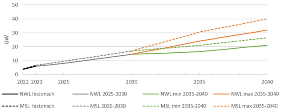
Abbildung 6: Hochrechnung Netzwerksame- und Modulsitzen-Leistung für Österreich, in GW (NWL = Netzwerksame Leistung; MSL = Modulsitzenleistung); Quelle: Eigene Erhebung und Hochrechnung
