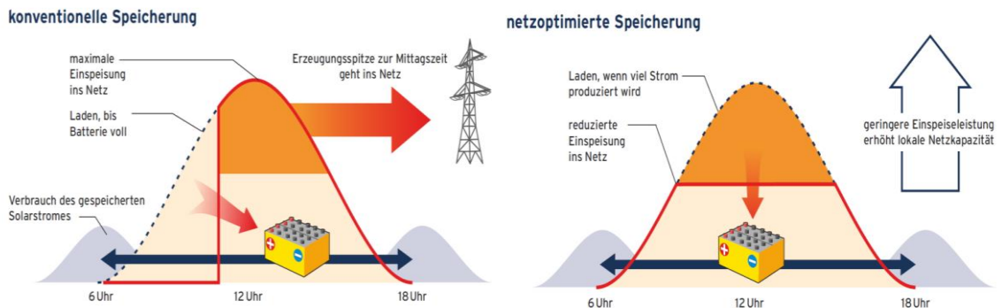
Abbildung 12: Netz- und marktoptimierte Speicherbewirtschaftung im Gegensatz zu einer konventionellen Speicherung [BSW 2013]
