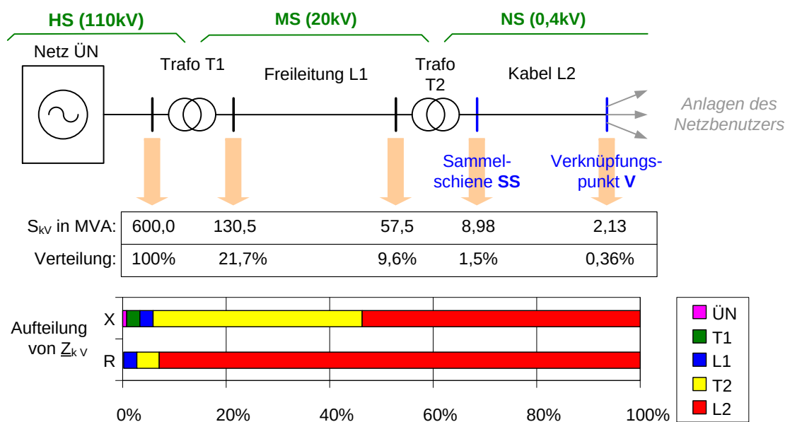
Abb. 3-1: Größenordnung der Kurzschlussleistungen und Anteile der einzelnen Netzelemente
