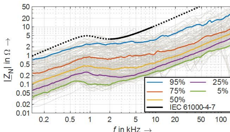
Abb. 6-3: Typische Verläufe der frequenzabhängigen Netzimpedanz (gemessen zwischen Leiter und Neutraleiter), gemessen in öffentlichen Niederspannungsnetzen in Deutschland, Österreich, der Schweiz und der Tschechischen Republik [9]
