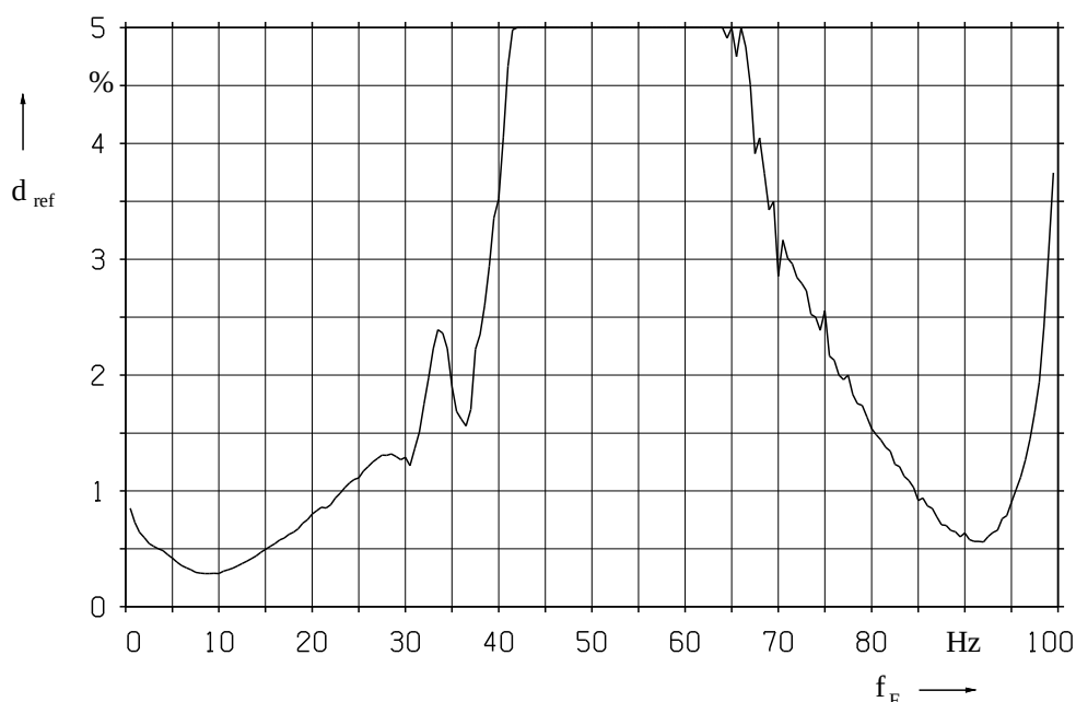
Abb. 4-4: Referenzkurve für P_{st} = 1 im Bereich bis f_F = 100 Hz ( r = 12000 \text{ min}^{-1} ) für rechteckförmige Spannungsschwankungen [2]
