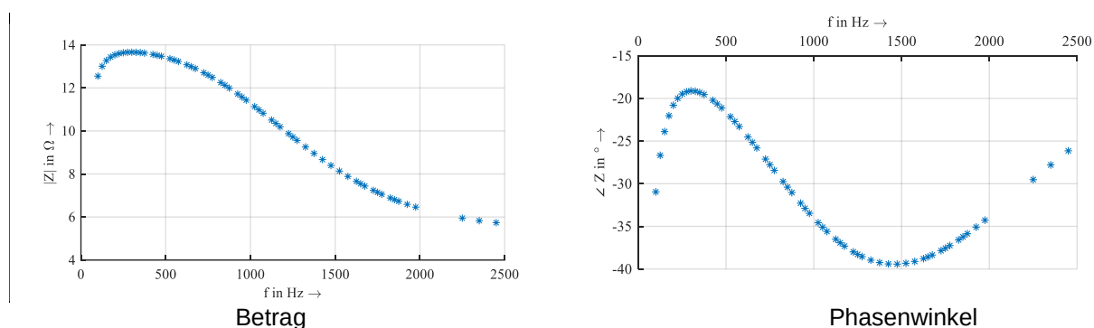
Abb. 6-1: Beispiel für Betrag und Phasenwinkel der frequenzabhängigen Eingangsimpedanz eines typischen On-Board Ladegleichrichters für Elektrofahrzeuge
