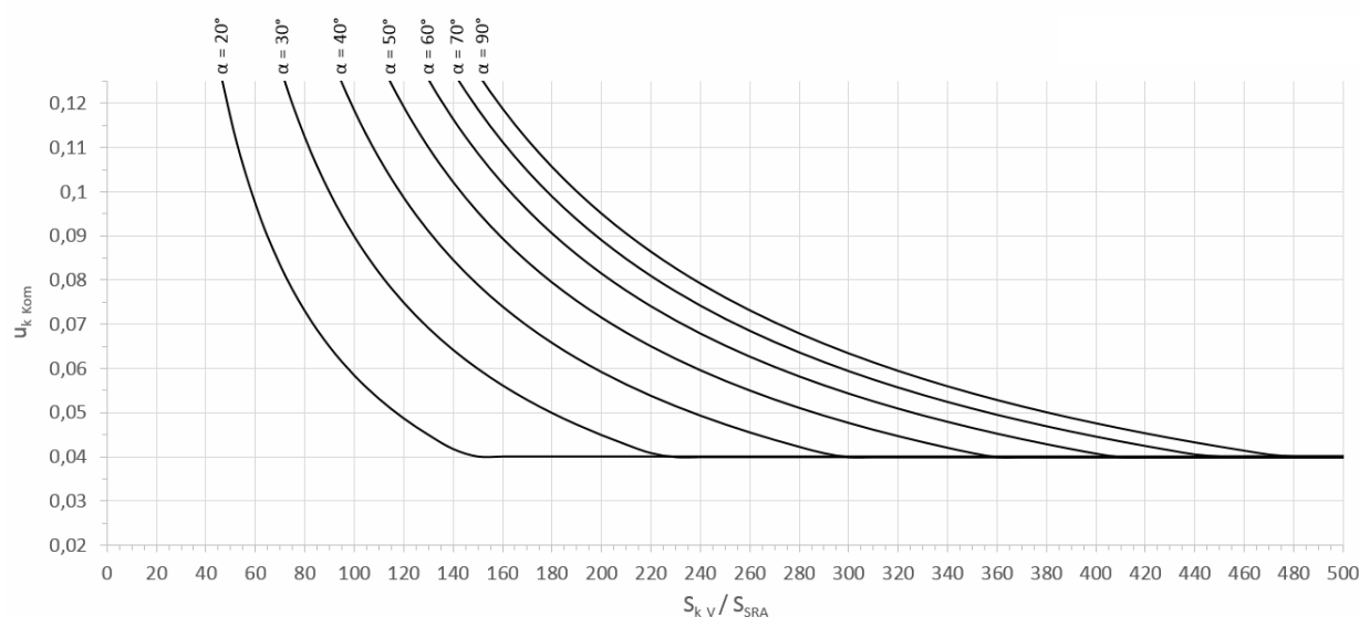
Abb. B-2: Erforderliche relative Kurzschlussspannung u_{k\,Kom} der Kommutierungsreaktanz X_{k\,Kom} in Abhängigkeit vom Verhältnis S_{k\,V} / S_{SRA} für verschiedene Steuerwinkel für 6-pulsige Stromrichter und d_{Kom} = 5\% (MS)
