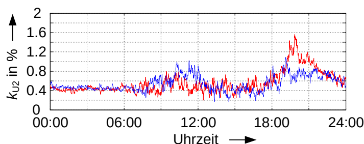
Abb. 5-1: Beispiel eines Tagesverlaufes des Unsymmetriegrads der Spannung in einem Netz mit (rot) / ohne (blau) einphasig ladende Elektrofahrzeuge [7]
