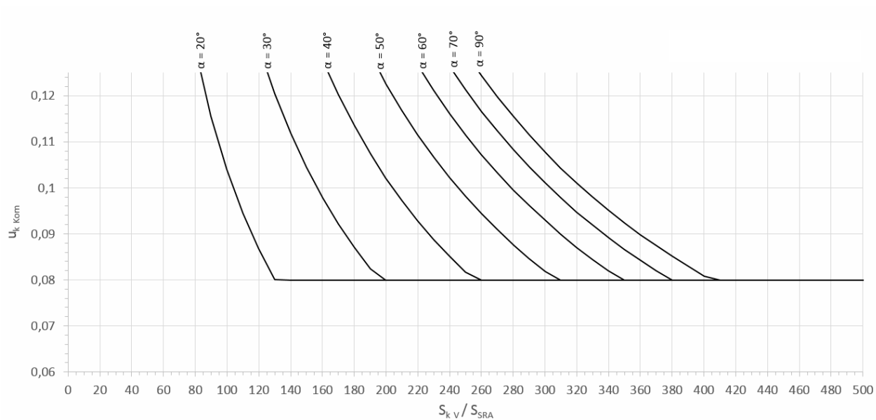
Abb. B-3: Erforderliche relative Kurzschlussspannung u_{k\text{ Kom}} der Kommutierungsreaktanz X_{k\text{ Kom}} in Abhängigkeit vom Verhältnis S_{k\text{ V}}/S_{\text{SRA}} für verschiedene Steuerwinkel für 6-pulsige Stromrichter und d_{\text{Kom}} = 3\% (HS)
