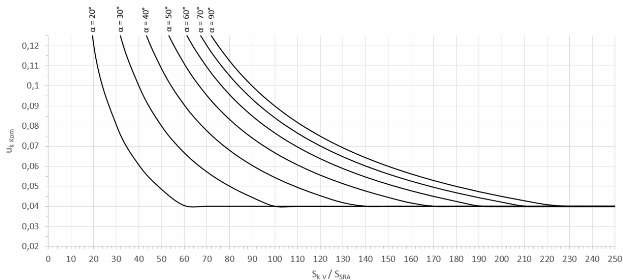
Abb. B-1: Erforderliche relative Kurzschlussspannung u_{k\,Kom} der Kommutierungsreaktanz X_{k\,Kom} in Abhängigkeit vom Verhältnis S_{k\,V} / S_{SRA} für verschiedene Steuerwinkel für 6-pulsige Stromrichter und d_{Kom} = 10\% (NS)
