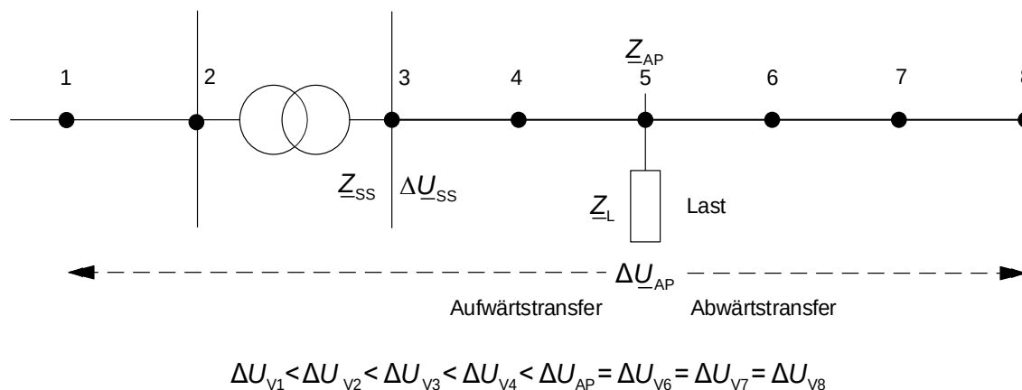
Abb. 4-10: Verteilung von Spannungsänderungen in einem strahlenförmigen Netz
