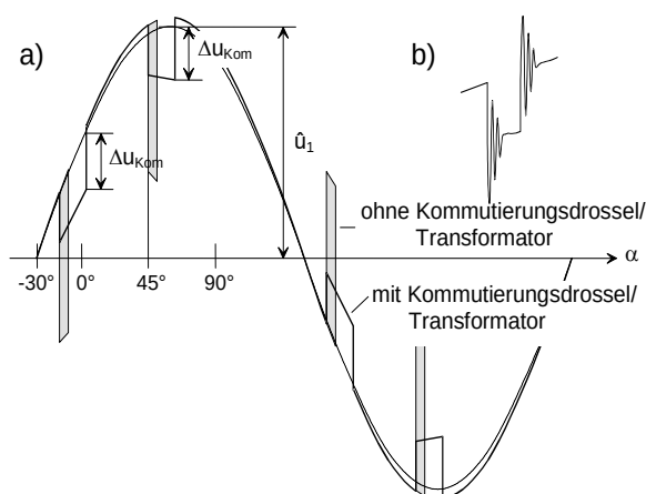
Abb. 7-1: Kommutierungseinbrüche in der Außen-/Neutralleiterspannung a) theoretischer Spannungsverlauf beim 6-pulsigen Stromrichter b) Einbruch mit Kommutierungsschwingungen (Detailausschnitt zu a)
